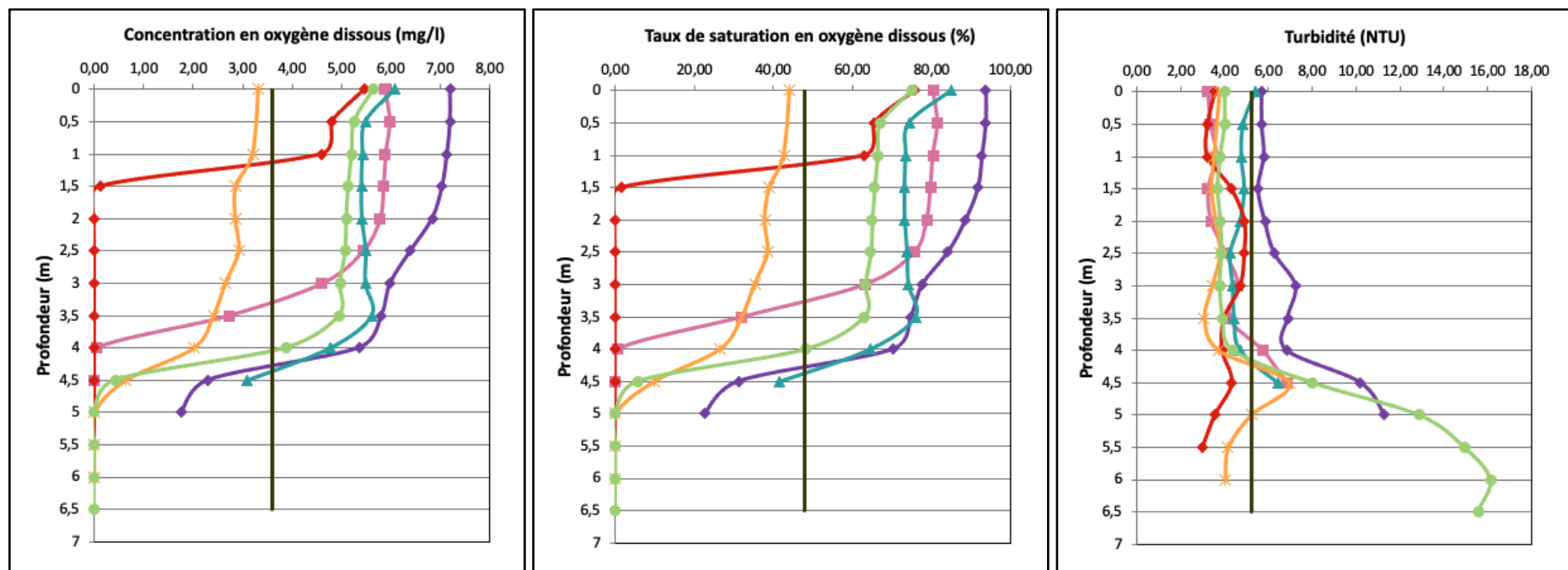
Figure 21 : Profils de la teneur en oxygène, de la saturation d'O 2 et de la turbidité en fonction de la profondeur pour les six campagnes de 2024 sur la retenue de Gaschet
