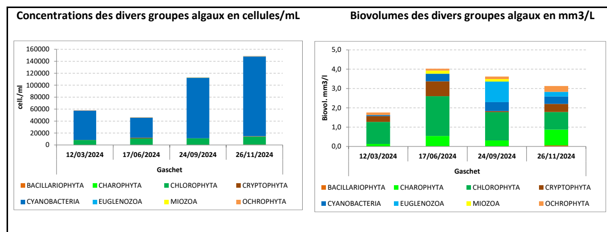
Figure 22 : Composition du peuplement phytoplanctonique pour la retenue de Gaschet en 2024 (Artémis)
