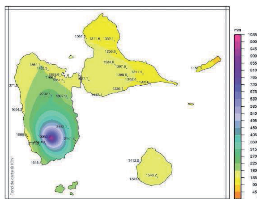
Figure 27: Précipitations moyennes annuelles entre 1981 et 2000
