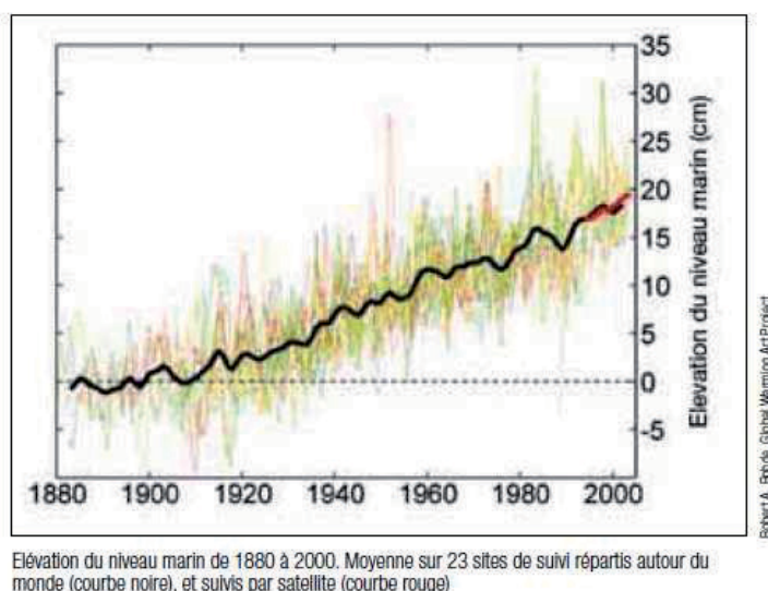
Figure 26: Élévation du niveau marin de 1880 à 2000
